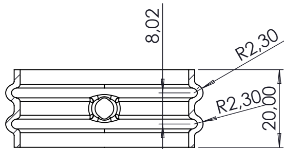
KESİT B-B ÖLÇEK 1 : 1
