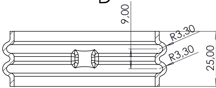
KESIT B-B ÖLÇEK 1 : 1
