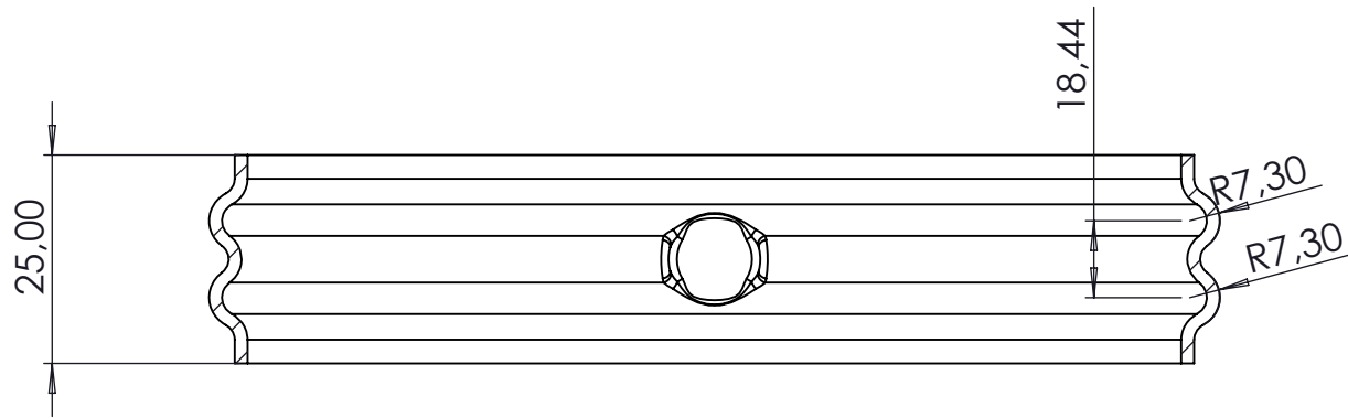
KESİT B-B ÖLÇEK 1 : 1
