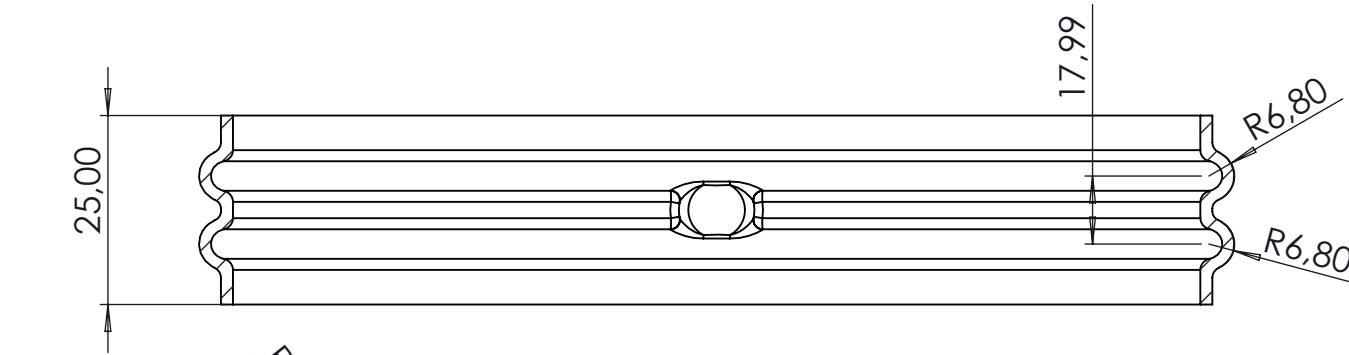
KESIT B-B ÖLÇEK 1 : 1
